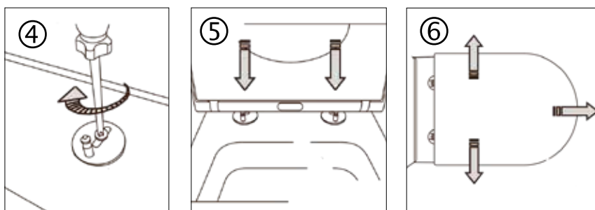
Fig. 4: Festebraketten med silikonpakning legges over plastlåsen og skrues delvis fast. NB! Velg korte eller lange skruer - det som passer til ditt toalett
