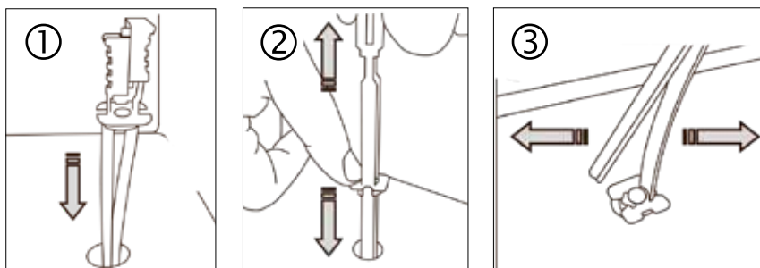
Fig. 1: Stripsankerets metallfeste settes i loddrett posisjon og skyves ned i monteringshullene på toalettet
